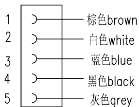
接线图 Circuit diagram
