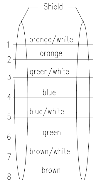
wiring diagram:
