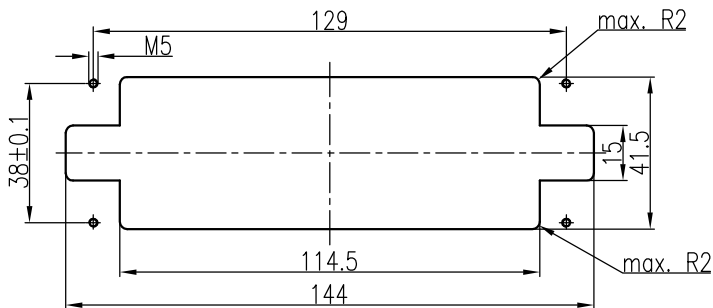
安装开孔图 Panel cut out
