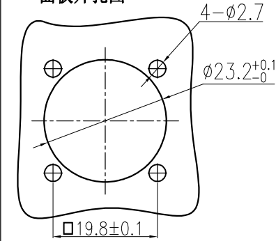
面板开孔图
