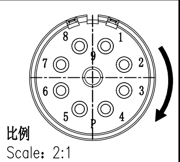
针位排布图
