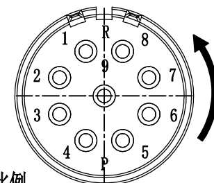
针位排布图
