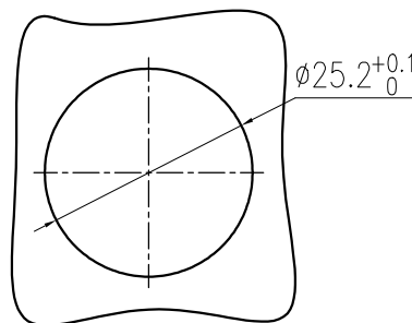
面板开孔图
