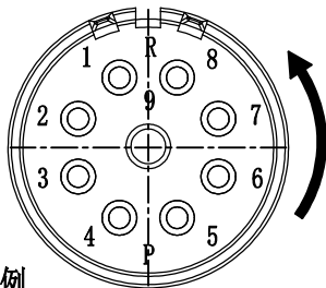
针位排布图
