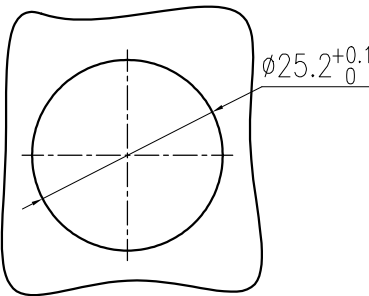
面板开孔图
