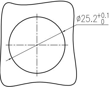
面板开孔图
