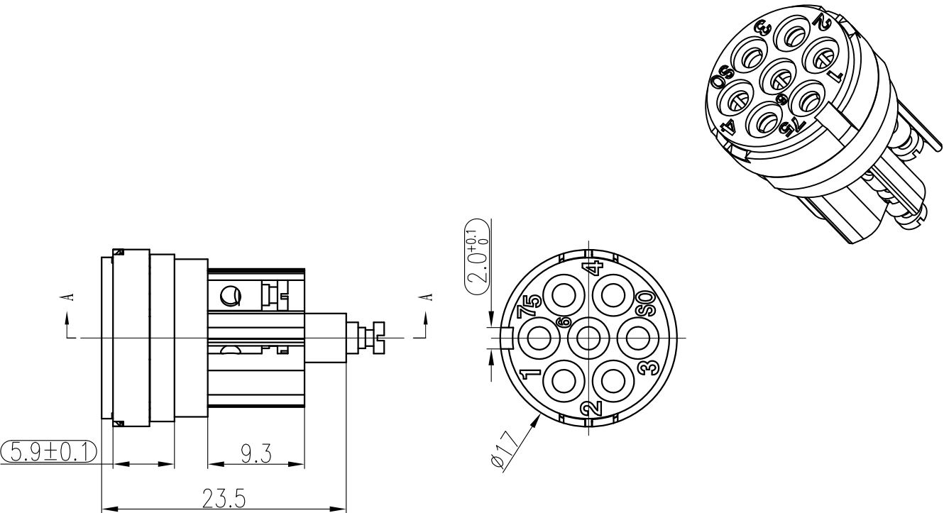
触点排列: 配合面 Contact arrangement: mating side
