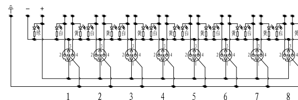
PNP回路
