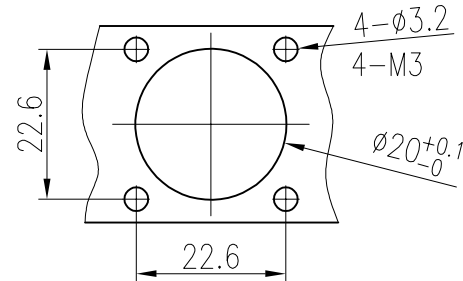
面板开孔尺寸图
