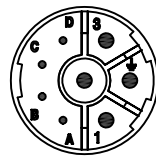
8(4+3+PE)
