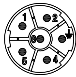
6(5+PE)
