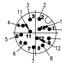
接线图 Circuit diagram
