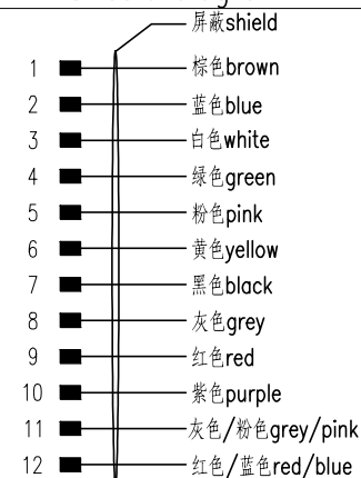
接线图 Circuit diagram
