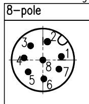
针位排布图
