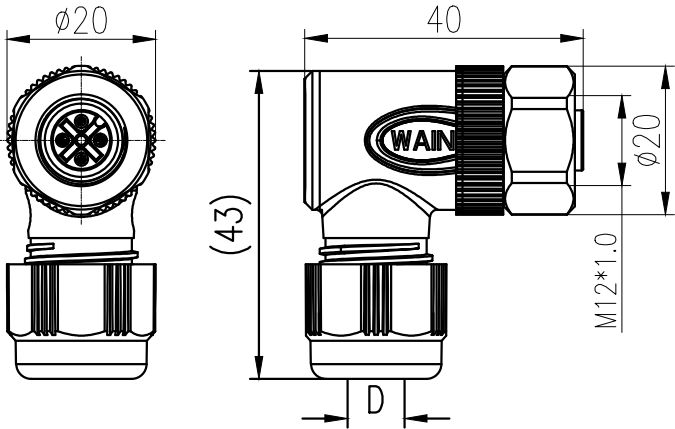
电缆直径:D6,D8 Cable outlet:D6,D8
