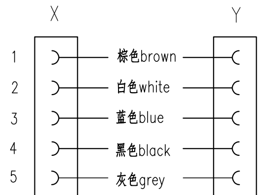
接线图 Circuit diagram
