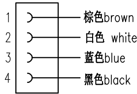
接线图 Circuit diagram
