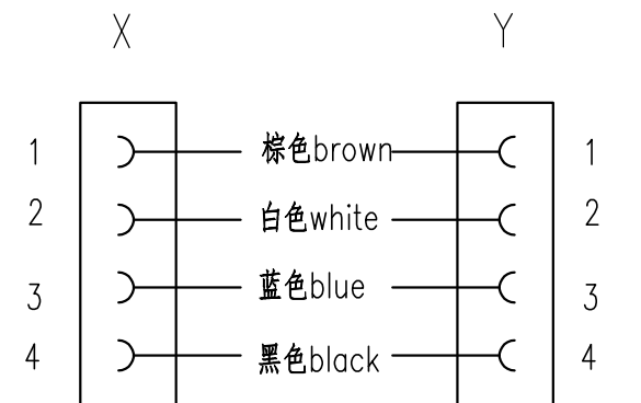
接线图 Circuit diagram
