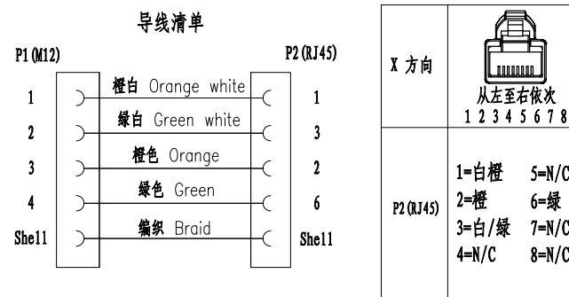
接线图 Circuit diagram
