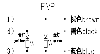
接线图 Circuit diagram
