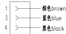
接线图 Circuit diagram
