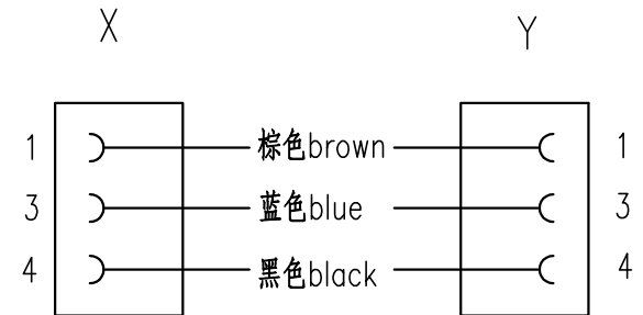
接线图 Circuit diagram
