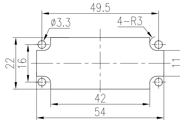
面板安装开孔图
