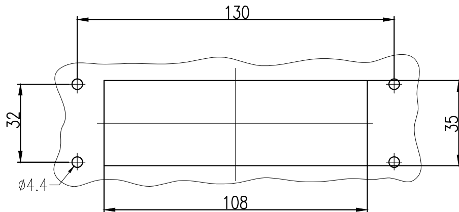
面板开孔图
