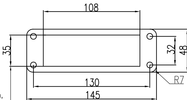
面板开孔图
