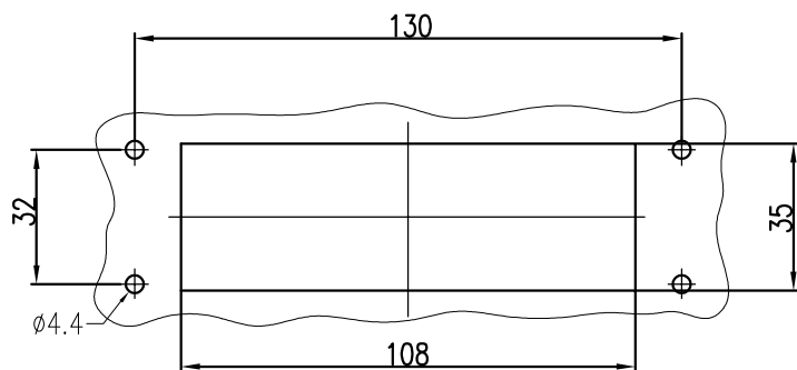
面板开孔图
