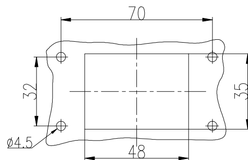
面板开孔图
