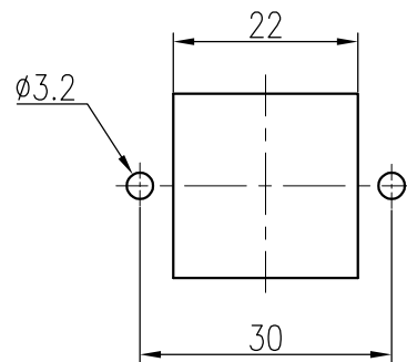
面板开孔图
