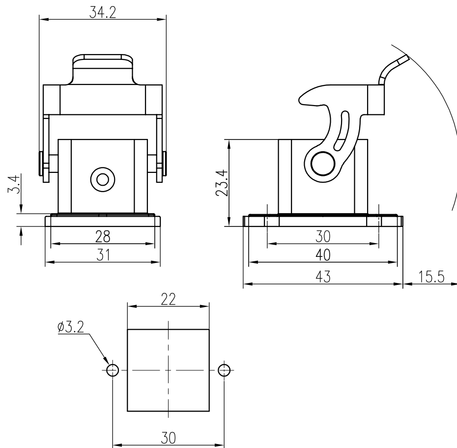
面板开孔图
