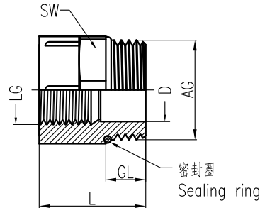
形式B Shape B
