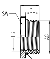
形式A Shape A
