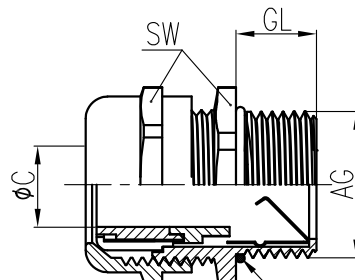
密封圈 Sealing ring
