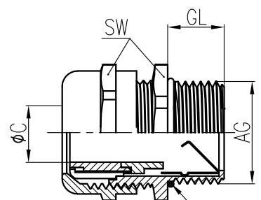
密封圈 Sealing ring
